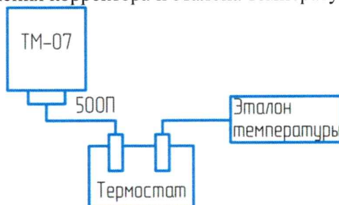
Рисунок 1 – Схема определение относительной погрешности измерения температуры
